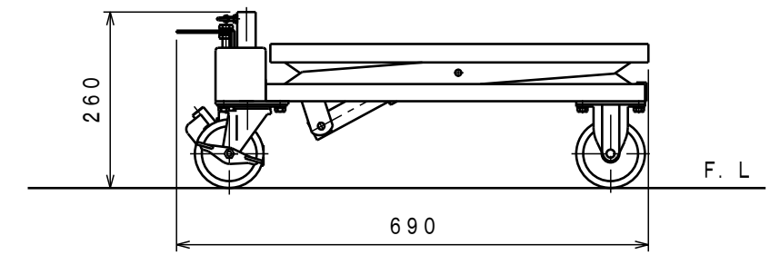
走行用ハンドル取り外し時外觀図
