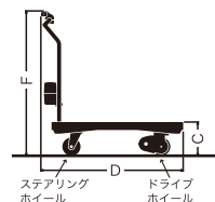
■寸法図(ASP-300-T2)
