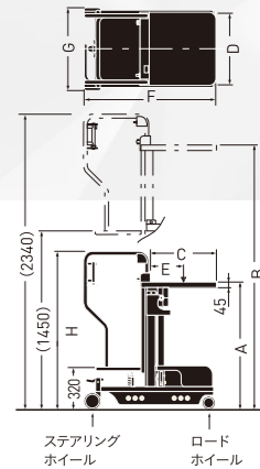
■寸法図 (サントピッカー)
