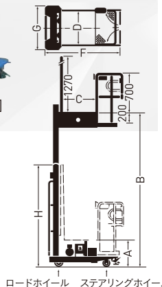
■寸法図 (ピッキングパワーリフター)
