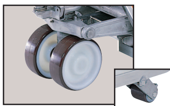
ウレタン車輪（ナイロン芯） ・ 標準タイプ（CP-10～25）に対応。
