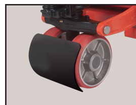
大車輪安全カバー 全機種に取付けできます。 注) パーキングブレーキとの併用は不可
