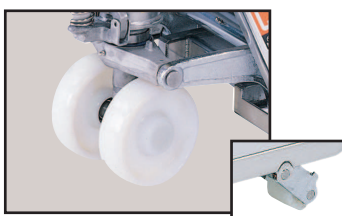
ナイロン車輪 ・ 標準タイプ（CP-10～25）に対応。
