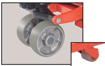
静電気拡散性車輪（アルミ芯） ・ 標準タイプ（CP-10～25）に対応。
