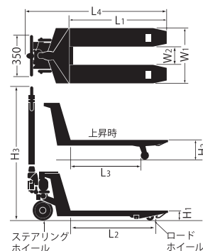
■寸法図（標準型・低床型）
