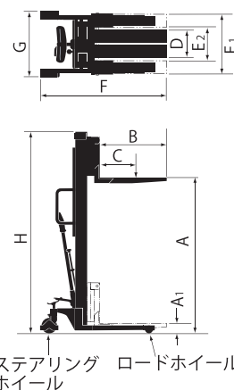
■寸法図（PL-H・PL-Dタイプ）
