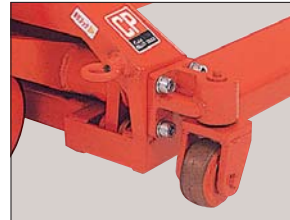
補助キャスター ●重量運搬専用型(5トン)用
